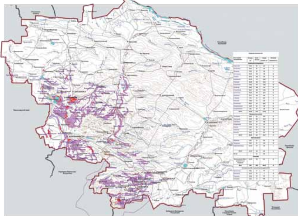
Схема потенциально-оползневых зон территории Ставропольского края
